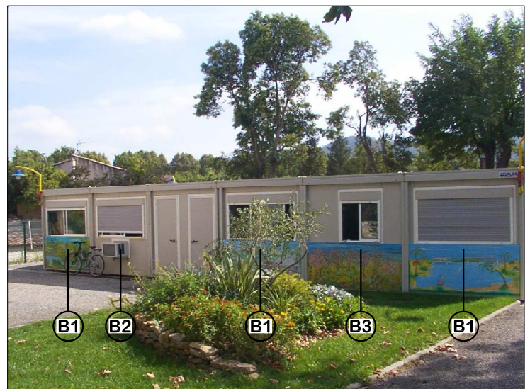
facade Nord - etat existant
